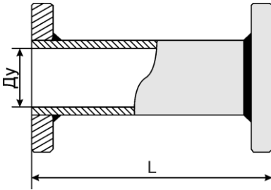
Габаритный имитатор ИПС Для ПРЭМ исполнения «сэндвич»
