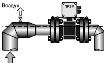
Рисунок 3 – Установка ПРЭМ в верхней точке трубопровода
